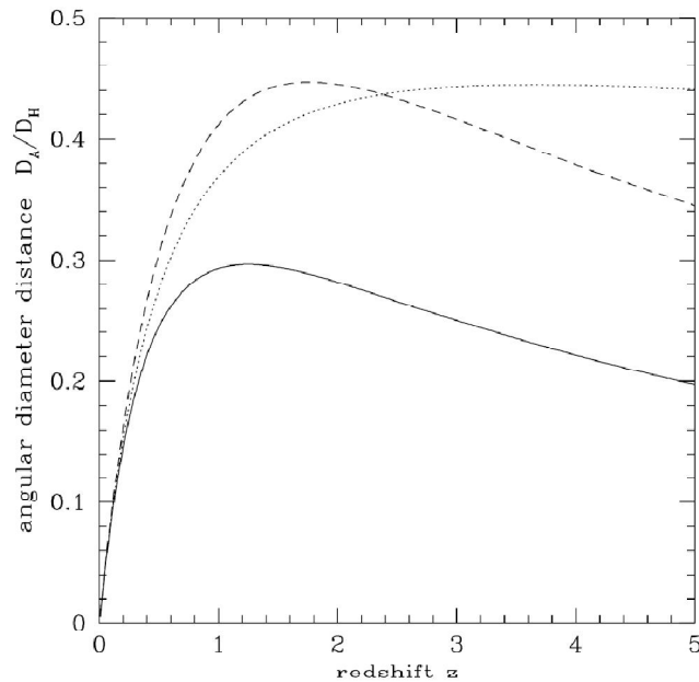
Рисунок 2: Безразмерное расстояние по угловому диаметру D_A/D_H . Три кривые отвечают трем моделям мира: Эйнштейна- де Ситтера (\Omega_M, \Omega_\Lambda) = (1, 0) , сплошная линия; с низкой плотностью (0.05, 0), пунктир; с большим значением лямбда (0.2, 0.8), штрих-пунктир.
